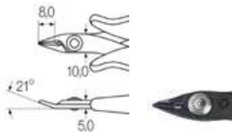
schmaler, spitzer Kopf und Drahthaltefeder ohne Wate Z 40 1 03
