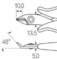
breiter, spitzer Kopf ohne Wate Z 46 0 03
