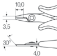
sehr schmaler, kurzer Kopf ohne Wate Z 46 0 03
