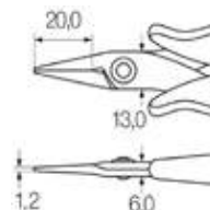
schmaler, kurzer Kopf gerade Form Z 36 0 03
